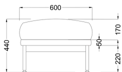
1.5 OTTOMAN DX-CPT-01S-BS 600(L) X 725(W) X 440(H)
