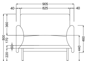
1.5 SEATER DX-CPT-1.5-SS 905(L) X 780(W) X 440(SH) X 800(H)
